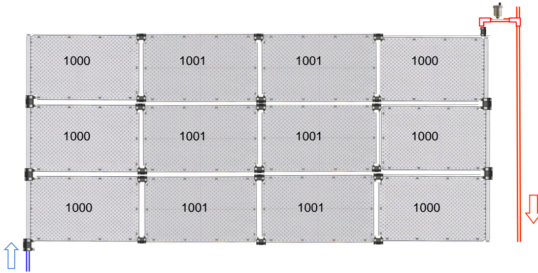
OKU-Absorber Art. N° 1000 und 1001 mehrere Reihen parallel waagrecht montiert
