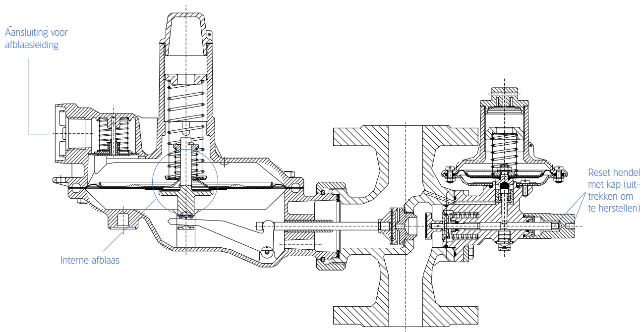
Fig.1: 133 regelaar met afslagveiligheid 033 en interne ontluchtingsklep
