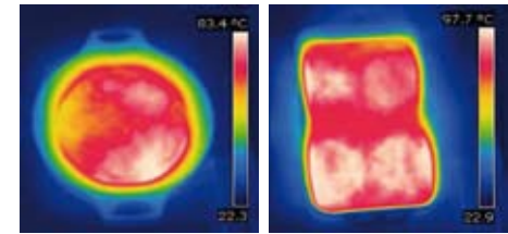
Distribución del calor en paellero circular
